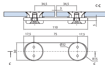
RA-011-S con tappo svasato RA-011-S with countersunk point RA-011-S mit versenkte Punkthalter
