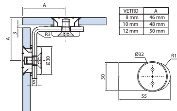
RA-011-S con tappo svasato RA-011-S with countersunk point RA-011-S mit versenkte Punkthalter
