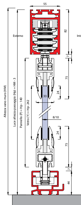
GUIDA ALLUMINIO INFERIORE ESTERNA
