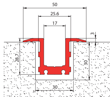
L-113 Canalina a terra alluminio Lavorazione pavimentazione Floor channel - Floor installation Bodenführung - Bodenvorbereitung
