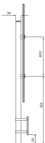
V-097 Attacco laterale per tubo corrimano Wall flange Wandflansch
