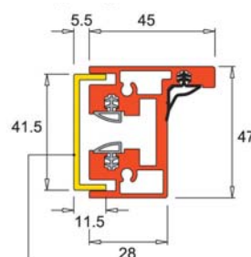
profilo a muro wall frame Wandprofil
