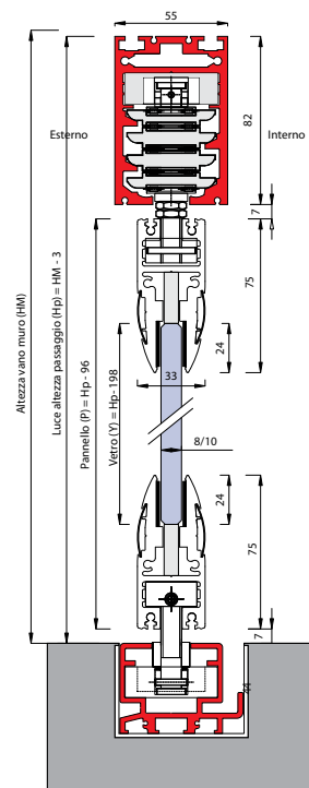
GUIDA ALLUMINIO INFERIORE INCASSATA
