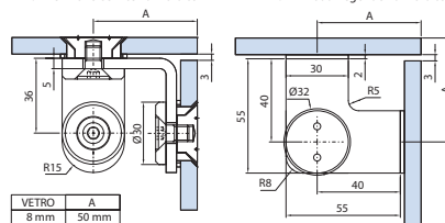
RA-011-S con tappo svasato RA-011-S with countersunk point RA-011-S mit versenkte Punkthalter
