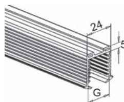
B-1015-21,5 GUARNIZIONE in caucciù per tubo scanalato per vetro 21,5 mm Rubber profile for channel tube for glass 21,5 mm Gummiprofil für Glasleistenrohr für Glas 21,5 mm
