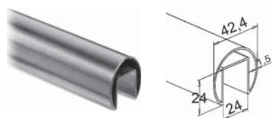
B-1010 TUBO PROFILO AD "U" scanalato Glass channel tube Glasleistenrohr
