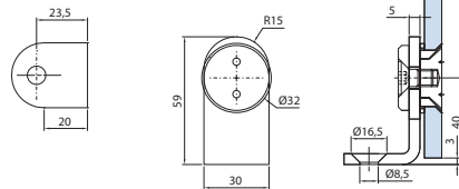
RA-011-S con tappo svasato RA-011-S with countersunk point RA-011-S mit versenkte Punkthalter
