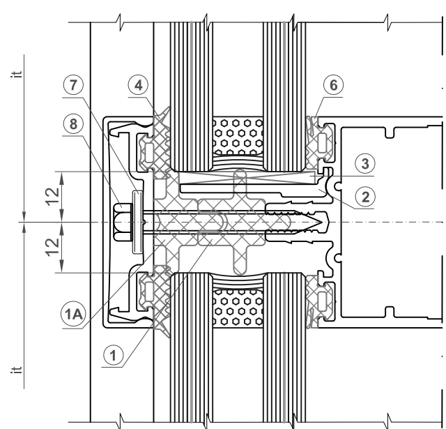
TRAVERSO
