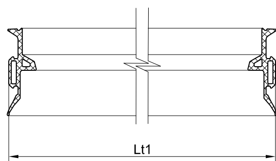
SEZ. AA :
