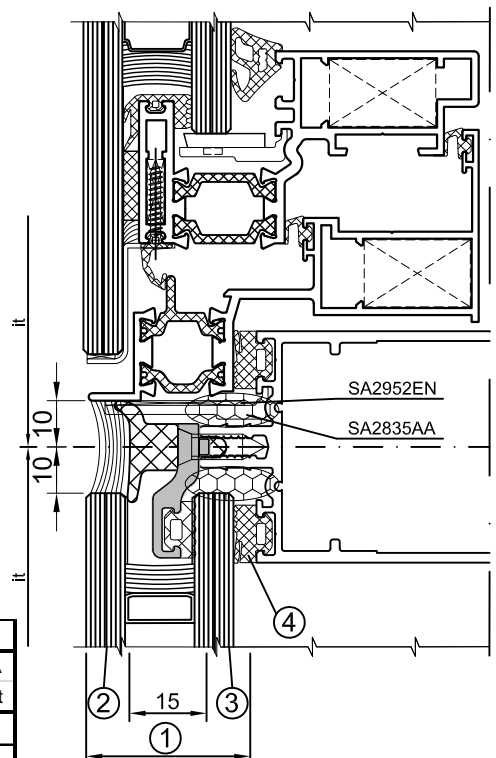
TRAVERSO - Transom
