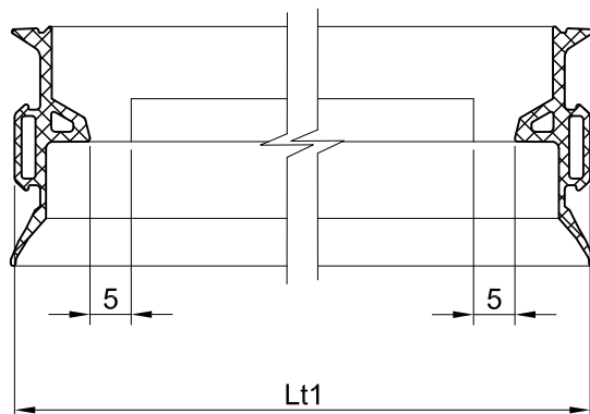
SEZ. AA :
