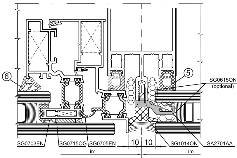
MONTANTE - Mullion
