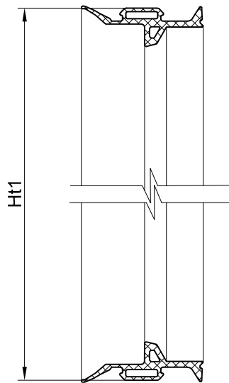
SEZ. BB :
