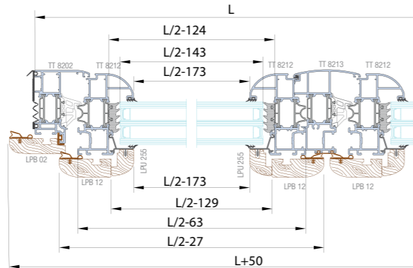
Sez. A-A
