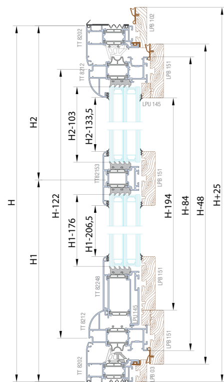
Sez. A-A
