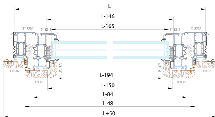
Sez. B-B
