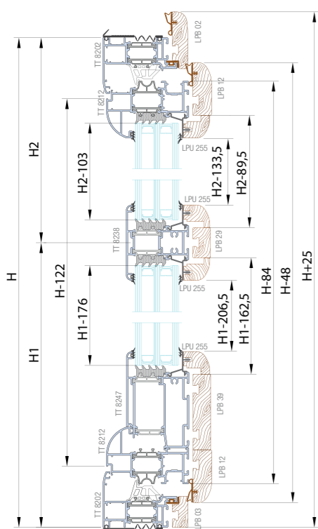
Sez. A-A
