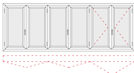
finestra 6 ante scorrevoli a libro 6 panel folding window
