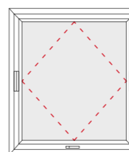
bilico orizzontale DIMENSIONI MINIME PER REALIZZARE UN SERRAMENTO BILICO CON CHIUSURA SU TUTTO IL PERIMETRO Hmin: 700mm Hmax: 2200mm Lmin: 576mm Lmax: 2950mm minimum dimension horizontal pivot window
