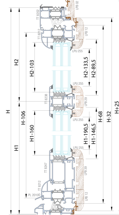
Sez. A-A
