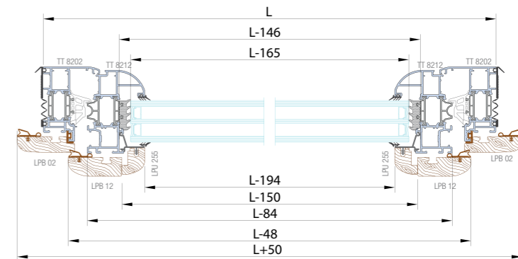
Sez. A-A
