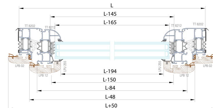
Sez. A-A
