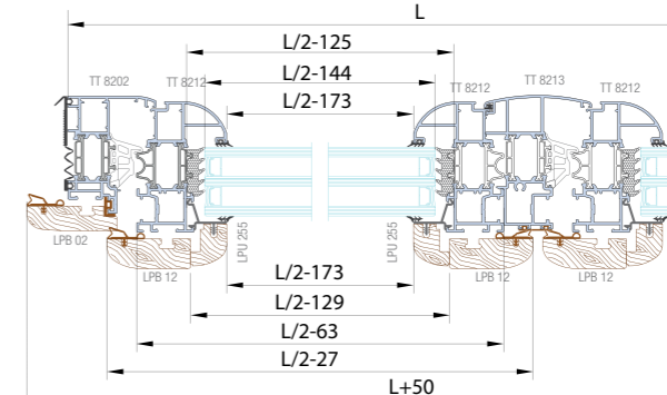
Sez. A-A
