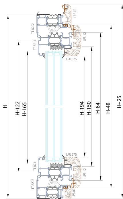
Sez. A-A
