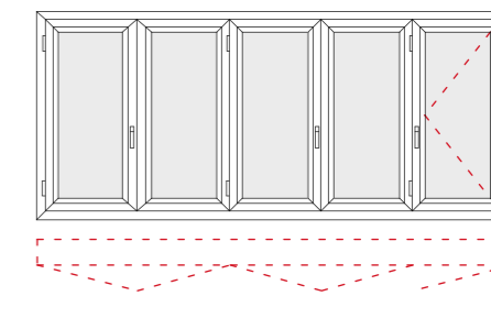
finestra 5 ante scorrevoli a libro 5 panel folding window
