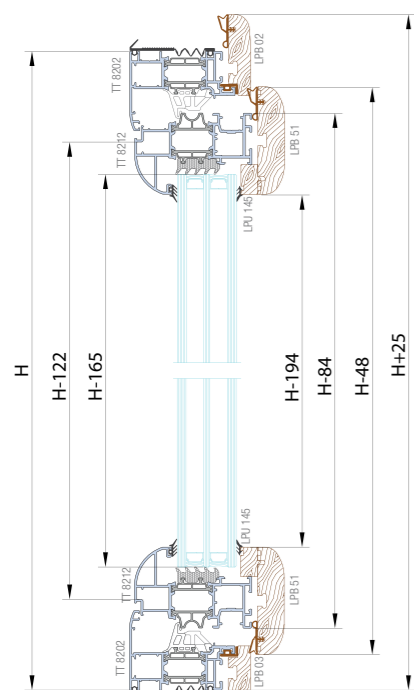
Sez. A-A
