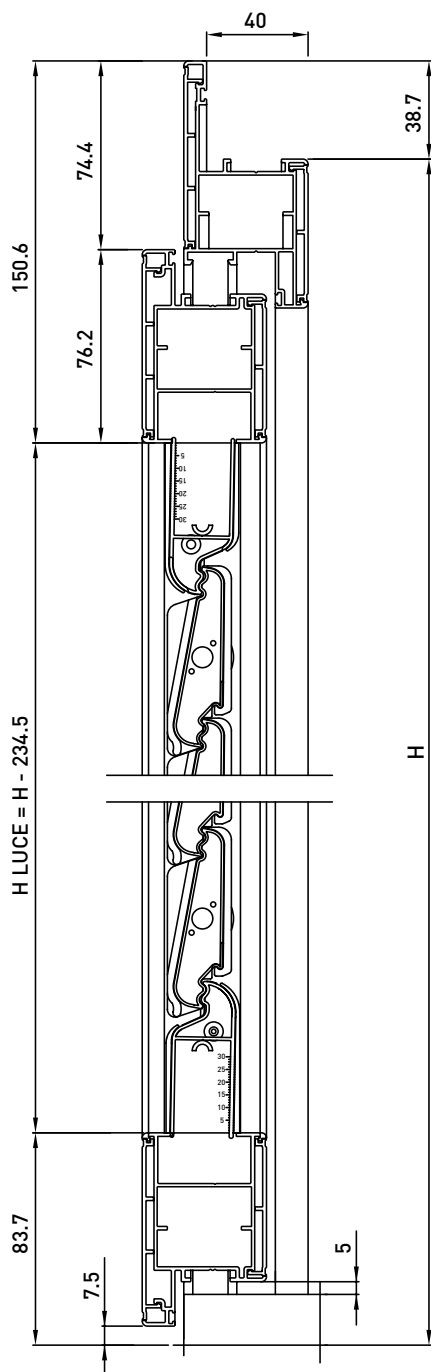
sezione B-B
