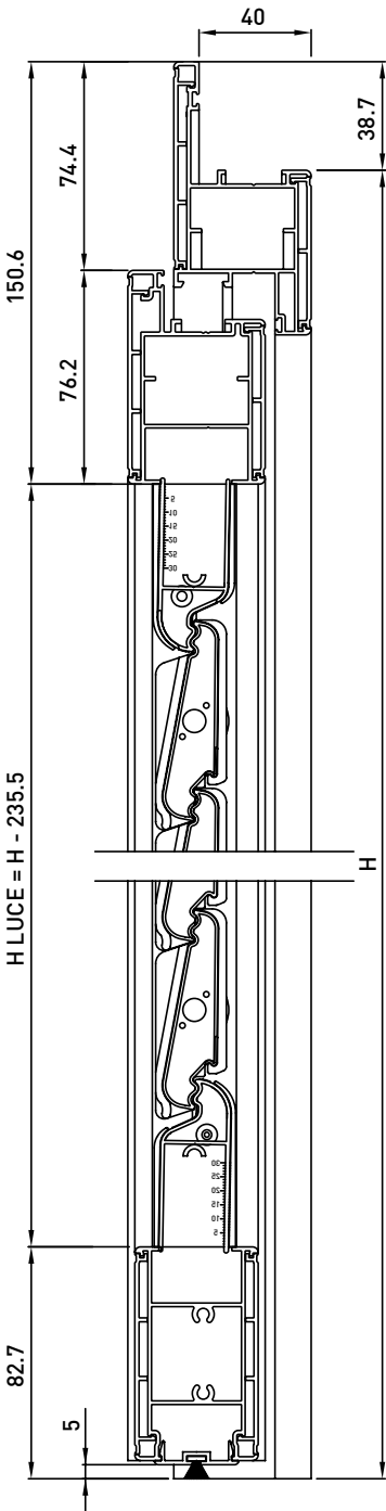
sezione A-A
