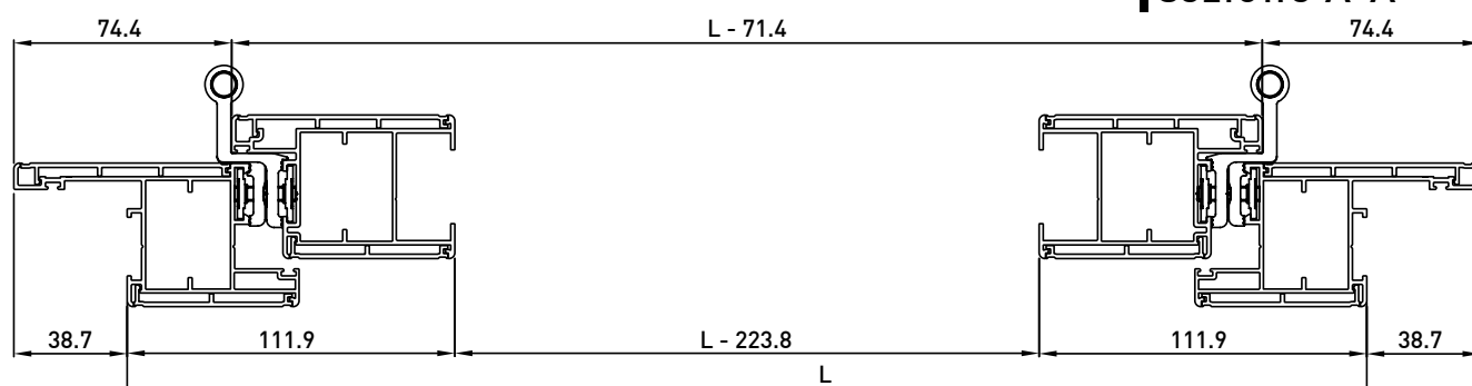
sezione A-A
