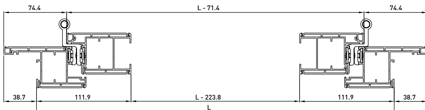
sezione A-A
