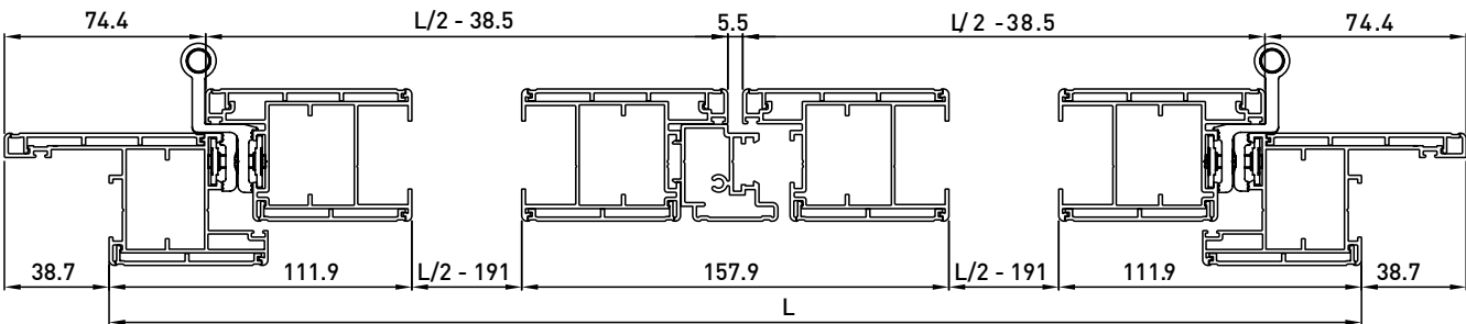
sezione A-A
