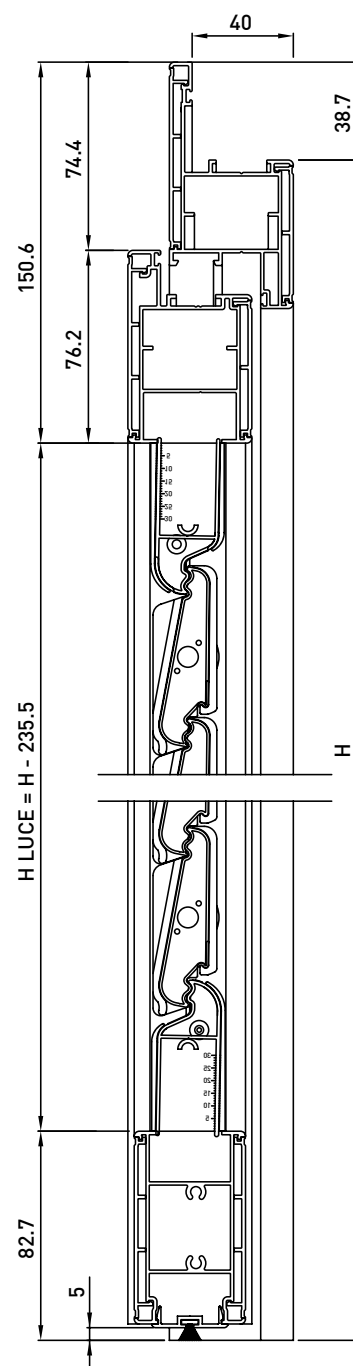
sezione A-A
