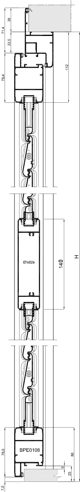
SEZIONE B-B
