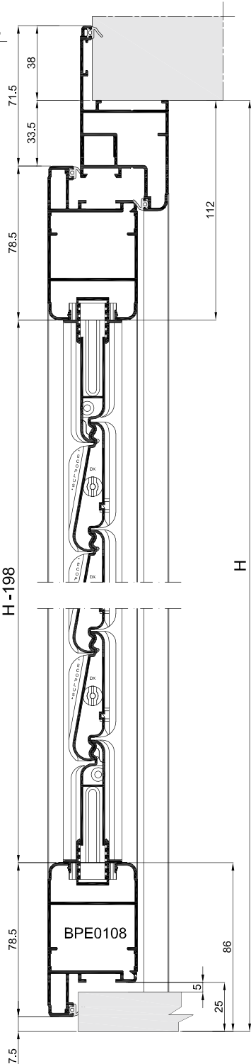
SEZIONE B-B
