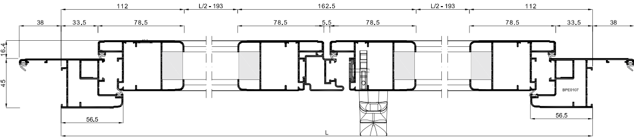
SEZIONE A-A
