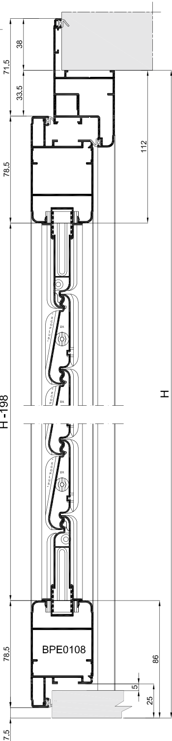
SEZIONE B-B
