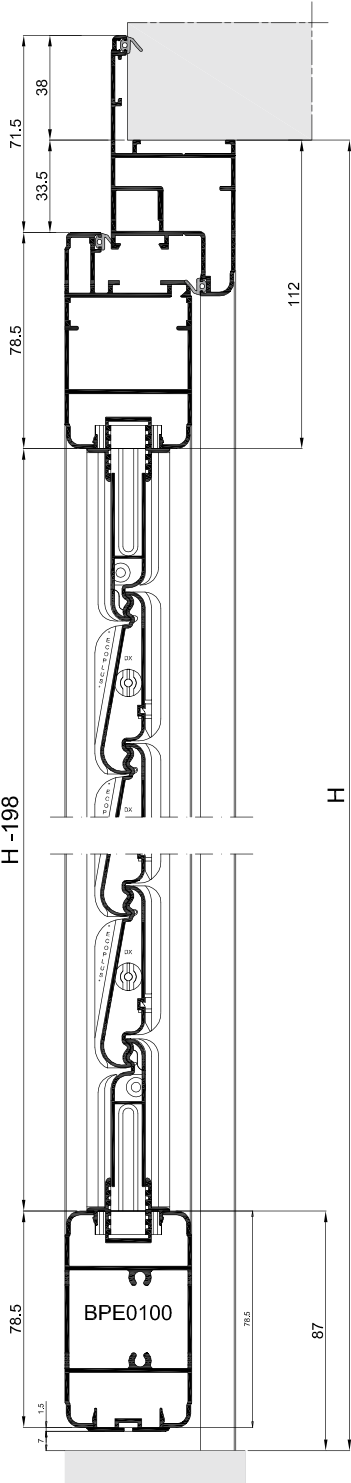
SEZIONE-BB
