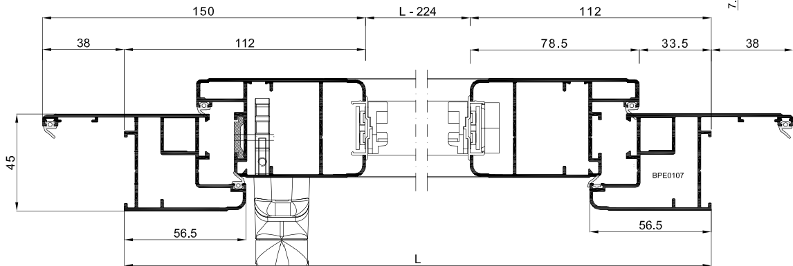
SEZIONE A-A
