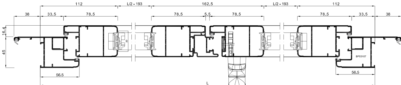
SEZIONE A-A
