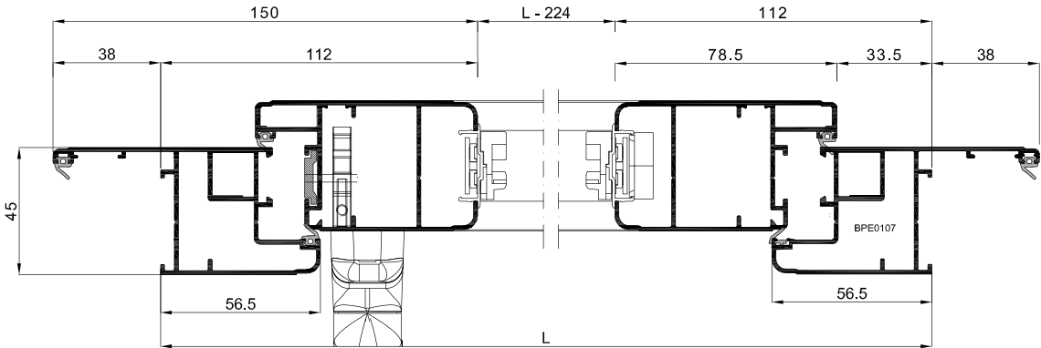
SEZIONE A-A
