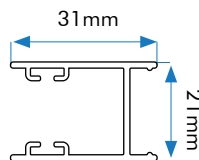
profilo ad "U" di compenso laterale
