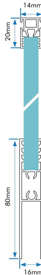
portavetro inferiore
