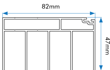
guida superiore a 4 vie
