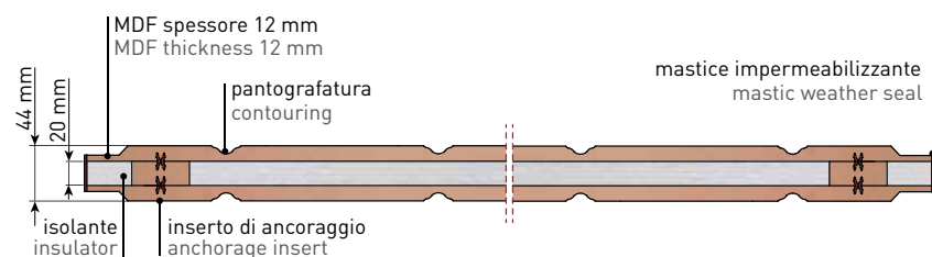
Sezione A-A | Section A-A
