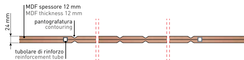
Sezione B-B | Section B-B
