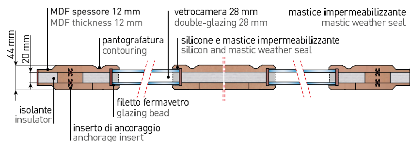
Sezione A-A | Section A-A
