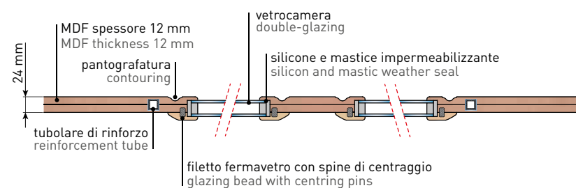
Sezione A-A | Section A-A
