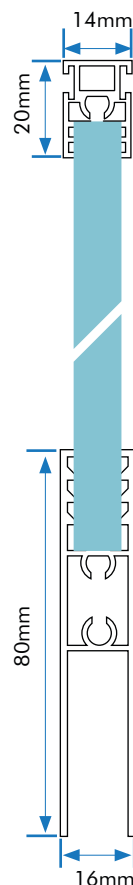
portavetro inferiore
