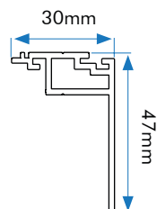
aggiunta guida superiore
