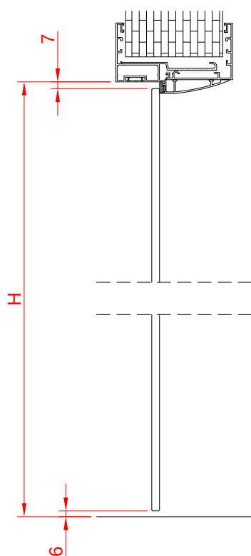
SEZIONE VERTICALE
