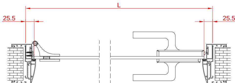
SEZIONE ORIZZONTALE
