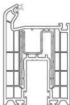
NUOVO RINFORZO
