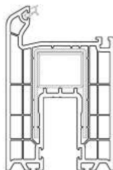
VECCHIA SOLUZIONE
