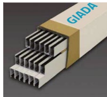
COD. V20308HS GUIDA ALTA 22x40 mm x 6.000 mm con SPAZZOLINO ANTIVENTO
