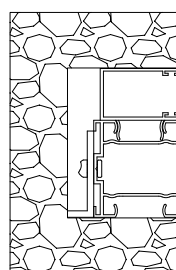
Sistema per tapparella da 70 mm
