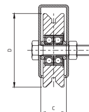
Ruota gola Y con scarico
