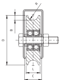
Ruota gola semitonda
