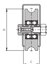
Ruota con ingrassatore gola semitonda
