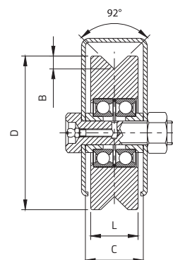
Ruota con ingrassatore gola V
