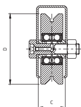
Ruota con ingrassatore gola Y
