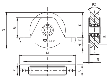
Ruota con supporto interno gola V
