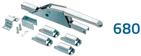
Carigione "Car" aste esterne 14x14 mm
