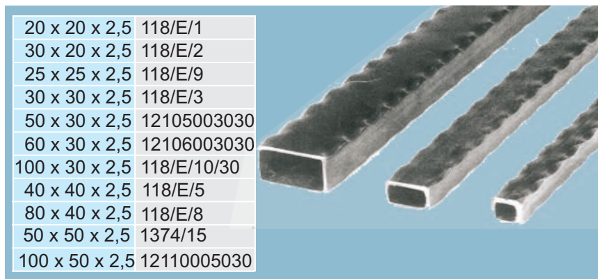
TUBO QUADRO E RETTANGOLO SPIGOLATO
